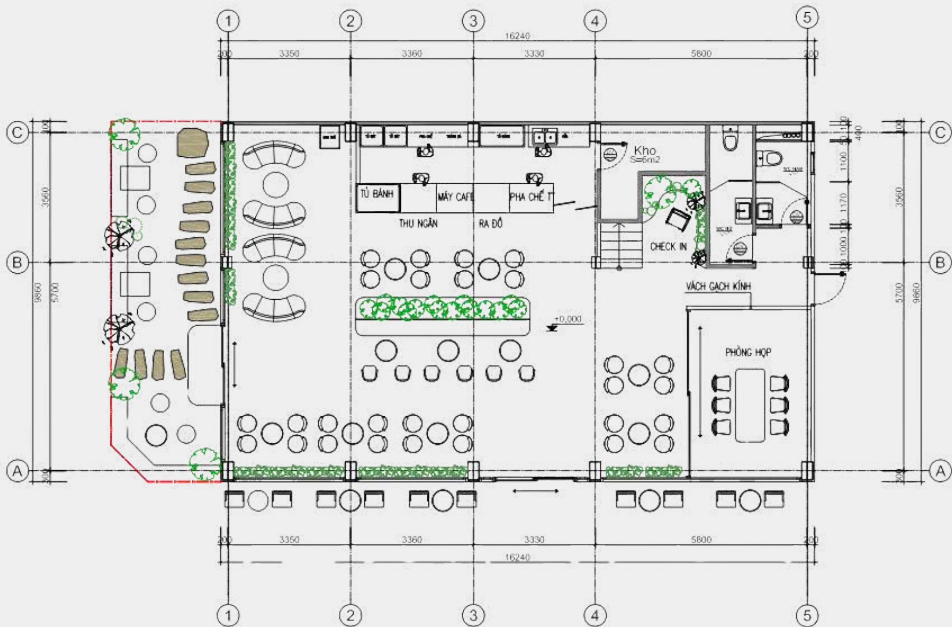
MẶT BẰNG NỘI THẤT TẦNG 1
