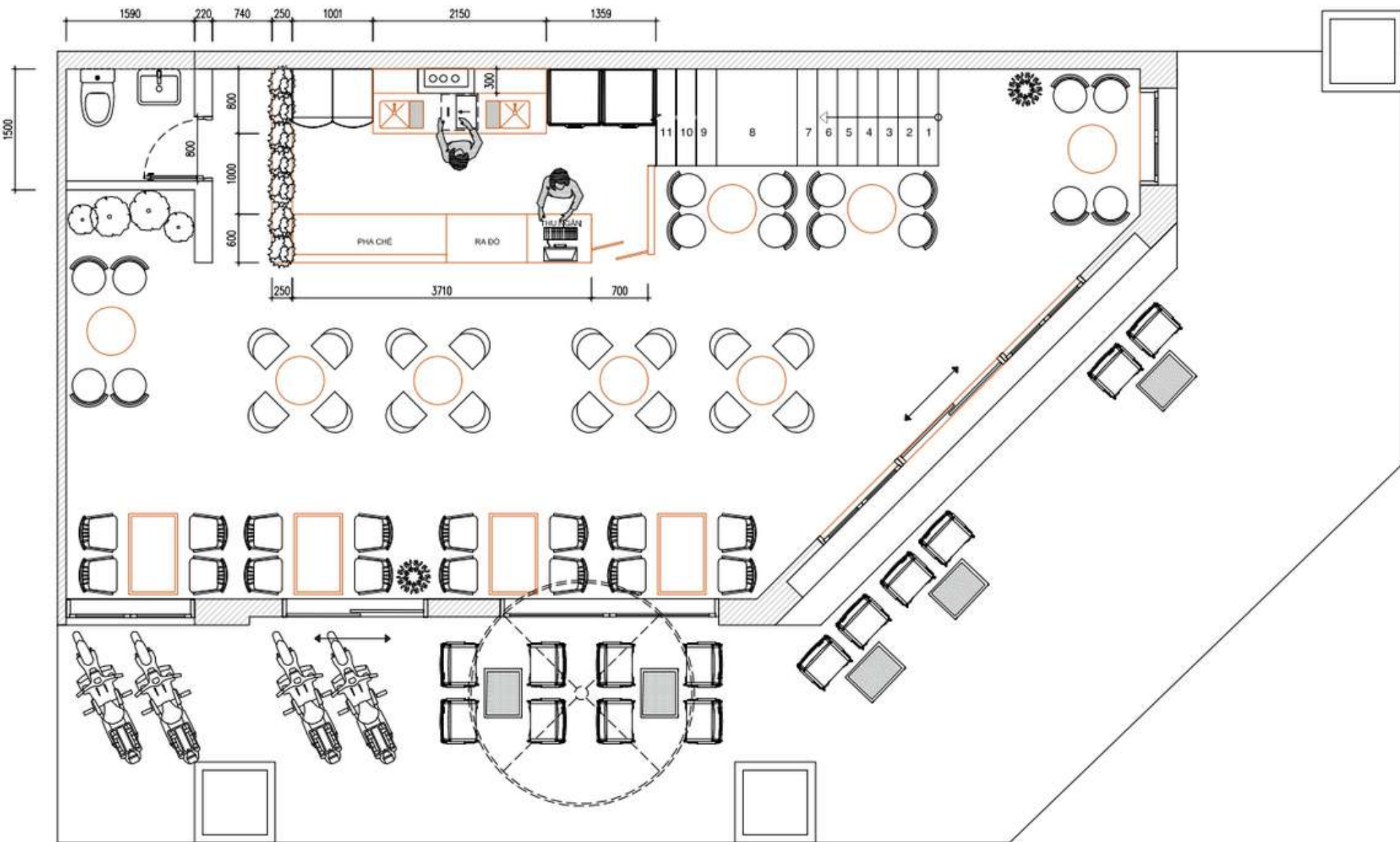
MẶT BẰNG NỘI THẤT TẦNG 1
